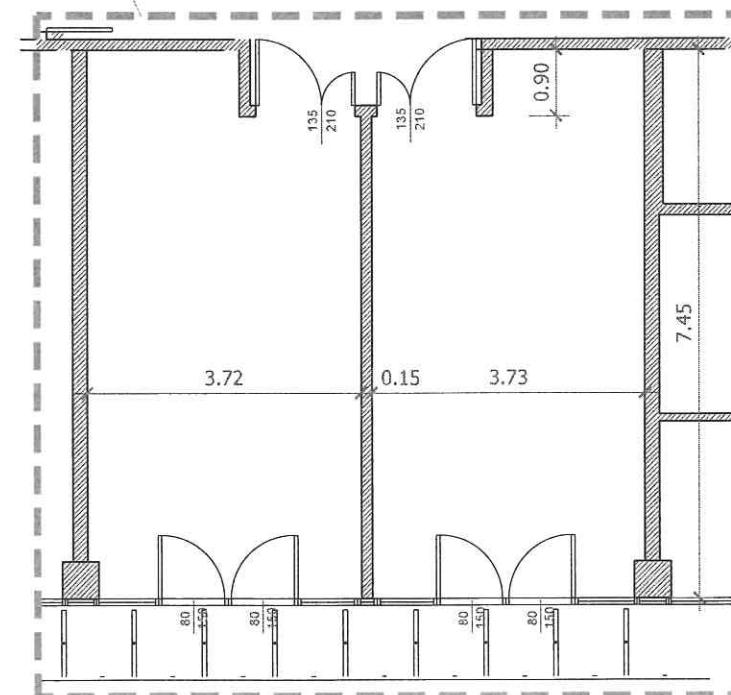
DETTAGLIO STANZA TIPO Scala 1:100
